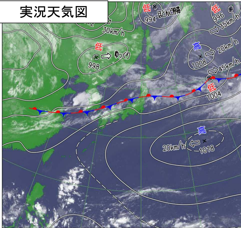
地上天気図 (7月10日6時)
