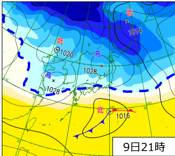
上空850hPa (約1500m付近)の気温
