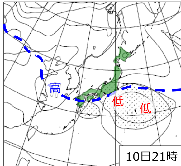
ハッチ域は、予想される24時間降水量が5mm以上の地域
